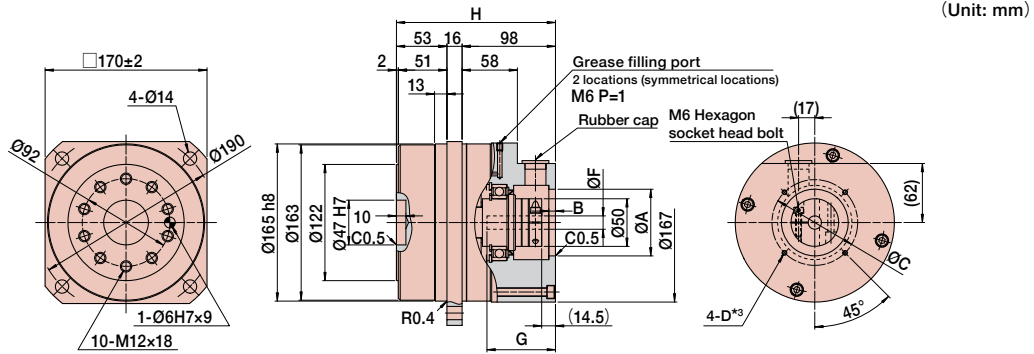
Flange Type I
